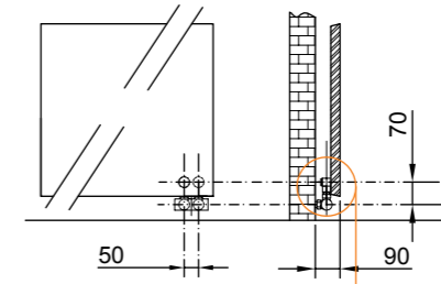
VALVOLA BITUBO
