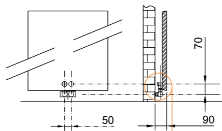
VALVOLA BITUBO
